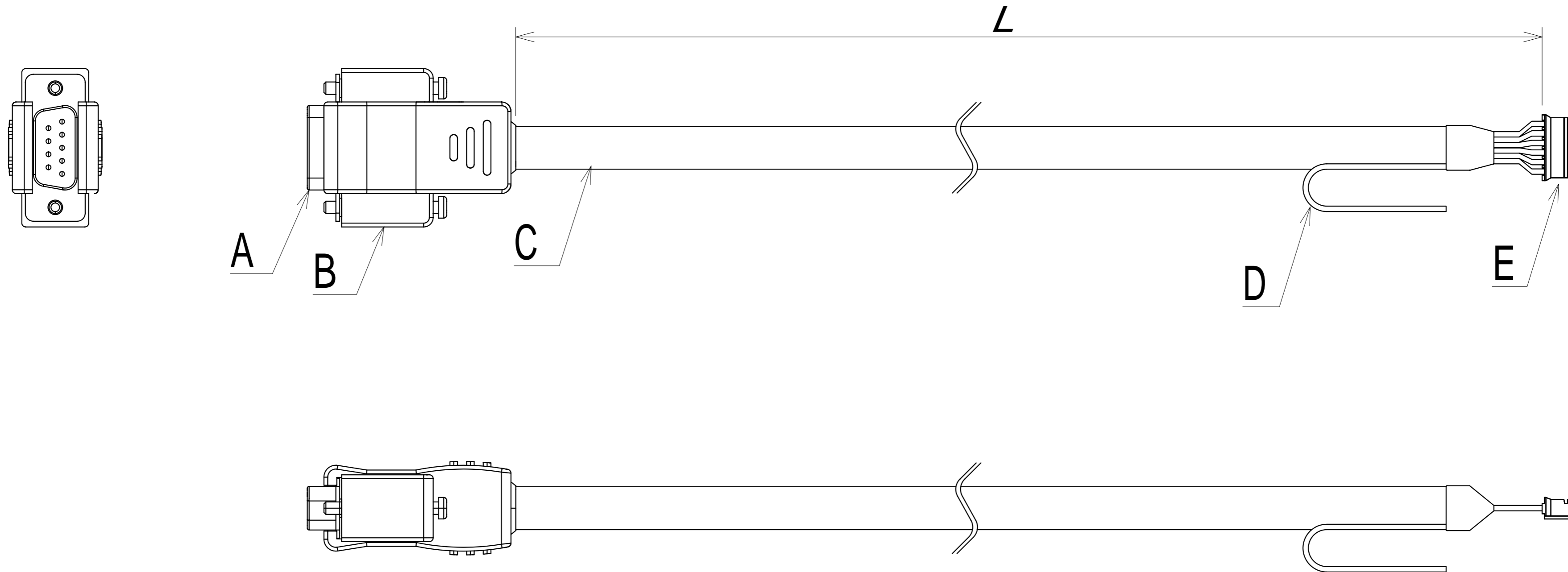
D-SUBコネクタ ピンアサイン
