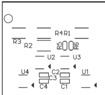
部品面
