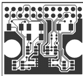
部品面
